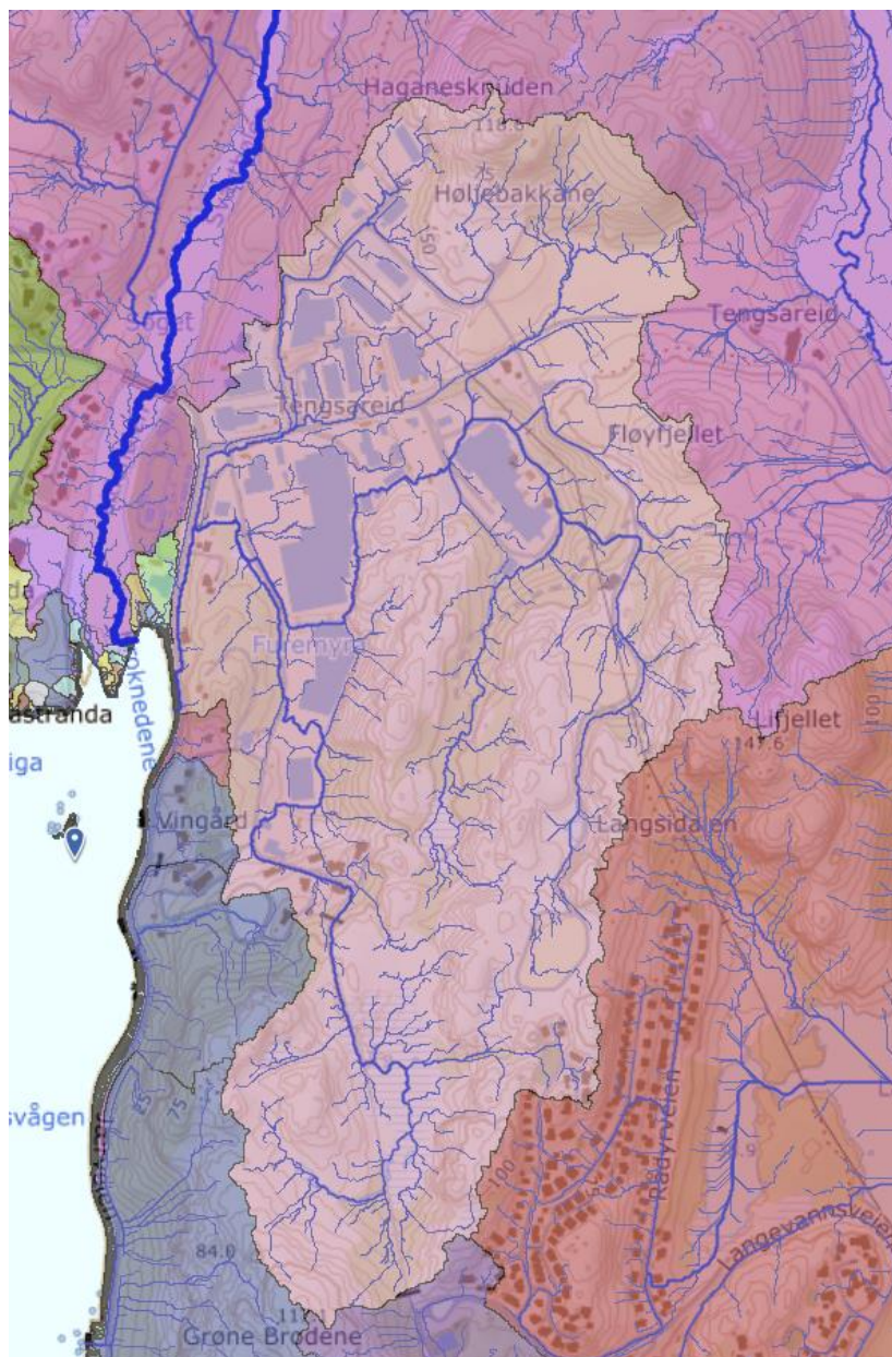
Figur 5 Eksisterende avrenning fra SCALGO Live.
