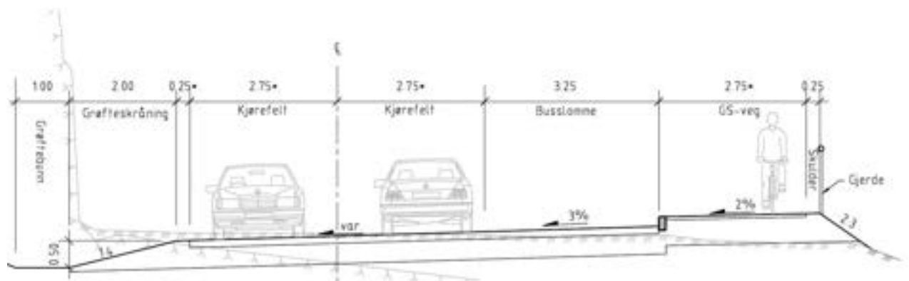
Figur 5-6 - Normalprofil Ytstebrødveien
