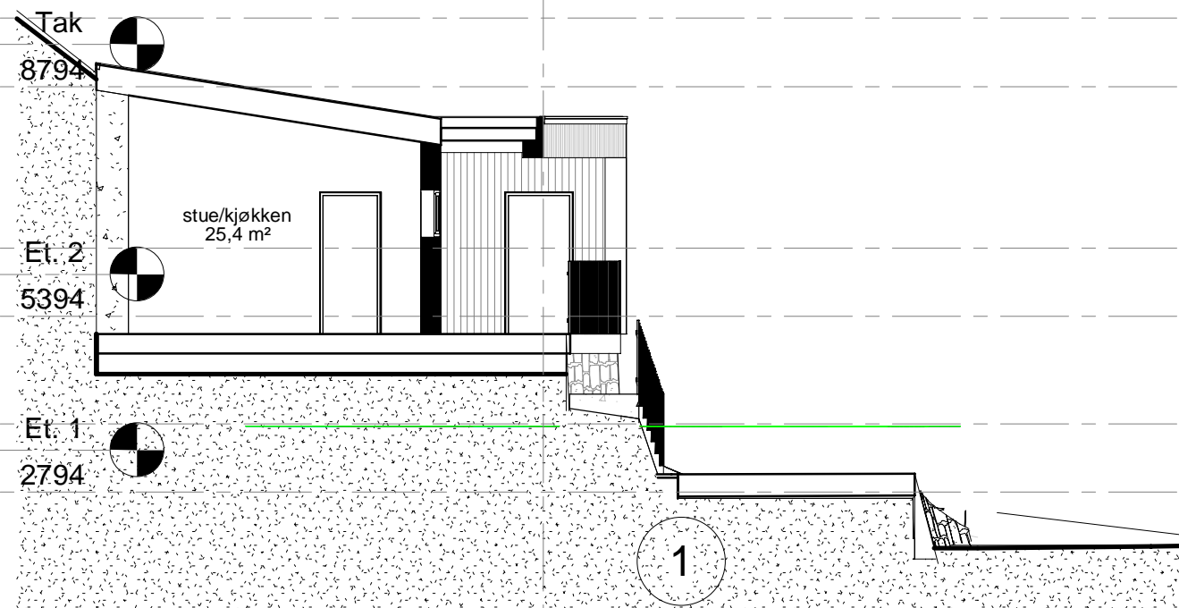
Snitt BB 1 : 100
