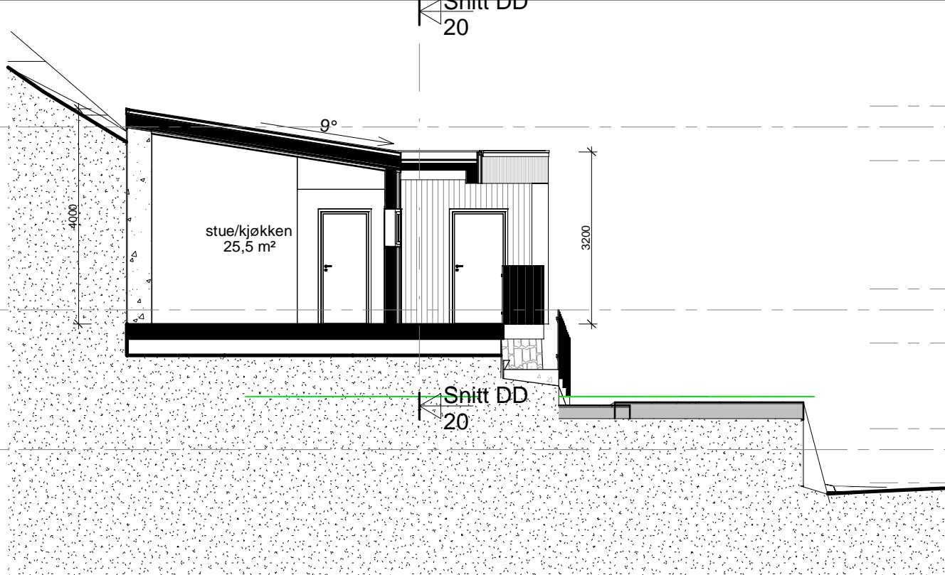
Snitt AA 1 : 100
