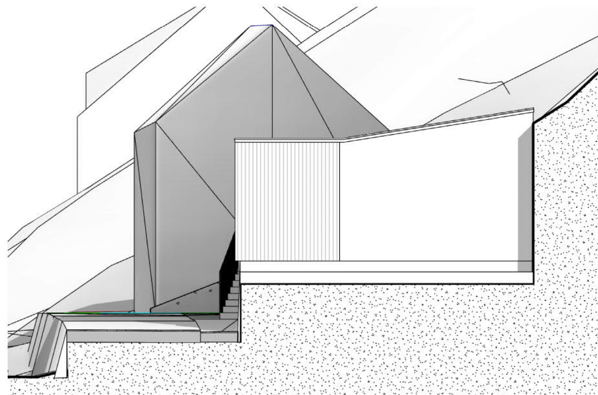
Øst 1 : 100
