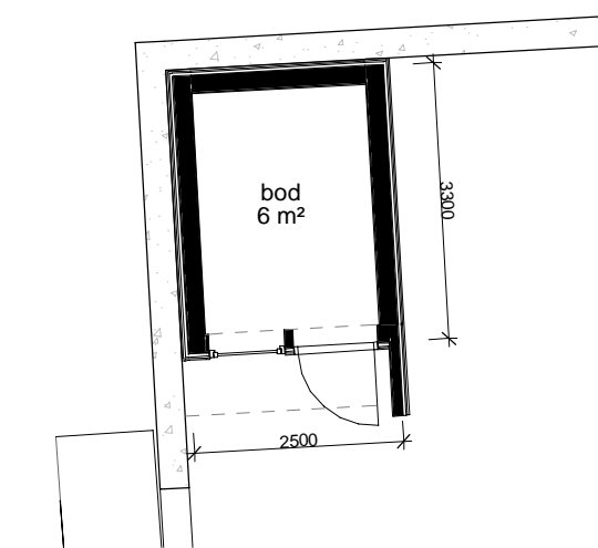
Bod 1 : 100
