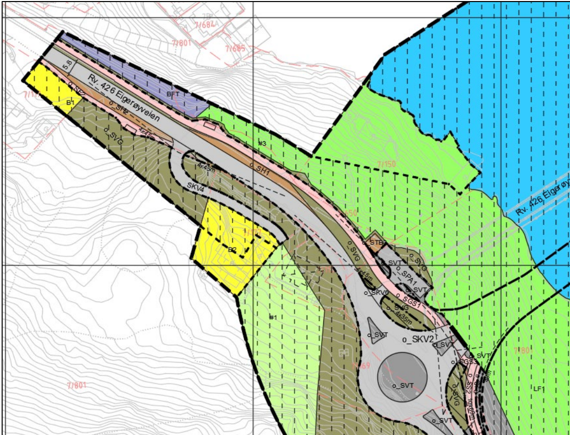
Figur 2 Utsnitt av gjeldende reguleringsplan ID 20220001 Ny eigerøy bru.
